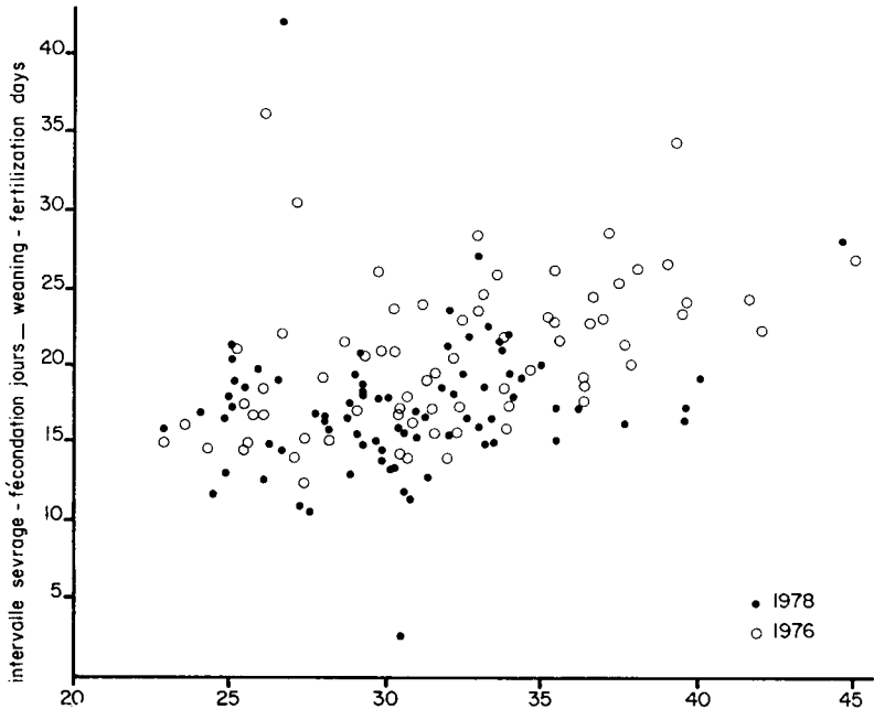
FIG. 4. — Relations entre la durée moyenne d'allaitement (x) et l'intervalle Sevrage-Fécondation (y) (2 moyennes anormales sont supprimées).
